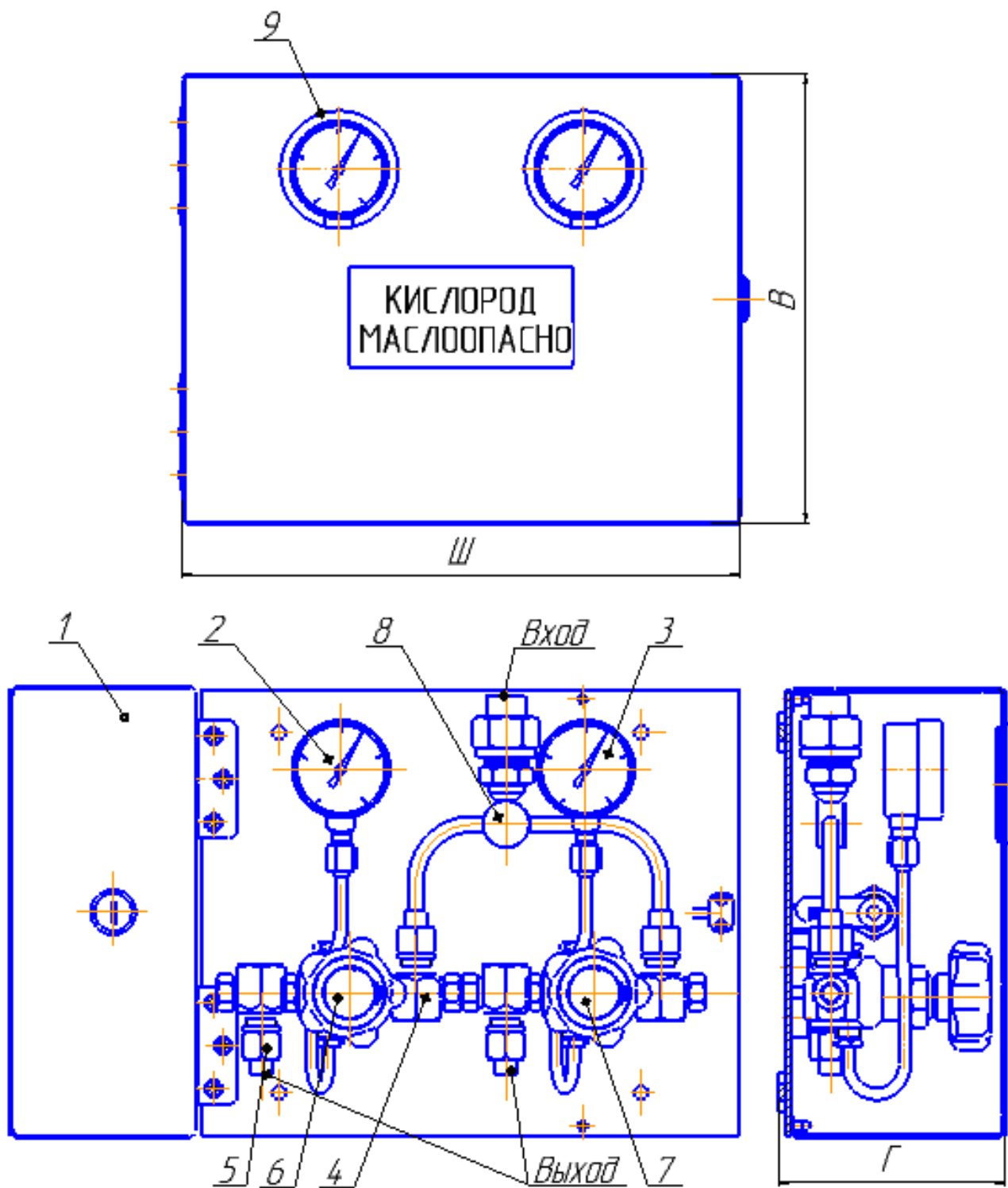
Рис.1 Поэтажная коробка ПК-4М(2x1)
